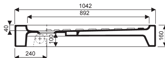
coupe AA' Receveur 007091 00 000
