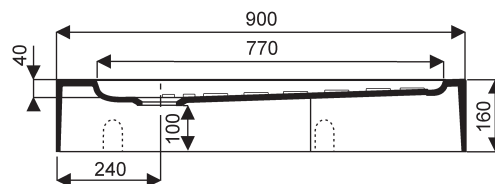
coupe AA' Receveur 007081 00 000
