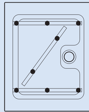
Implantation des pieds, receveur de 100 x 80
