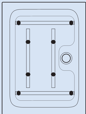
Implantation des pieds, receveur de 120 x 90
